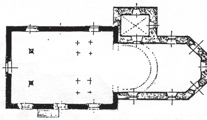
Grundriss nach der Wiederherstellung von 1686
